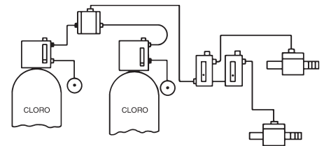
Modelo HYDRO 202-2 (T o W)* Reserva Automática con Múltiples Puntos de Alimentación
