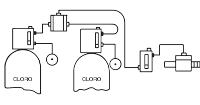
Modelo HYDRO 202 (T o W)* Reserva Automática
